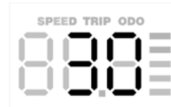
Kod błędu
